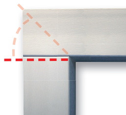
Het FRISIAN® kozijn heeft geen standaard schuine hoekverbinding maar een authentieke hoekverbinding van 90 graden.
