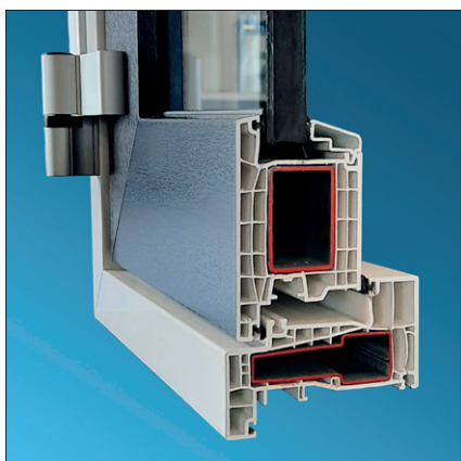
Extra zware staalversterkingen
